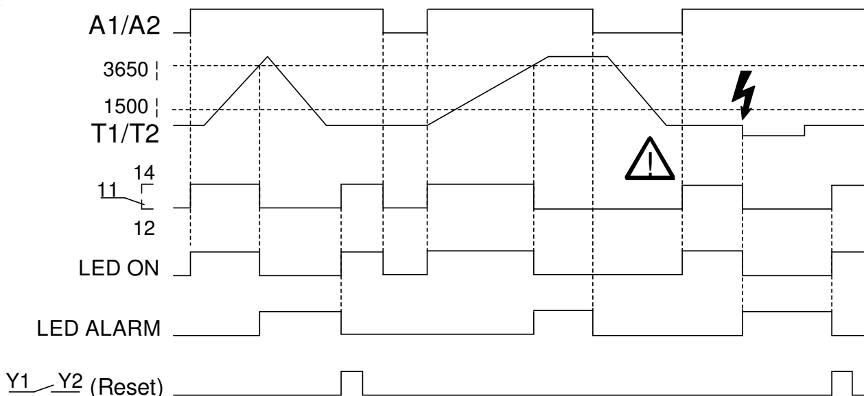
MSR 220 VA
